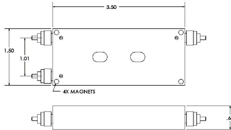
NoTail™ package
